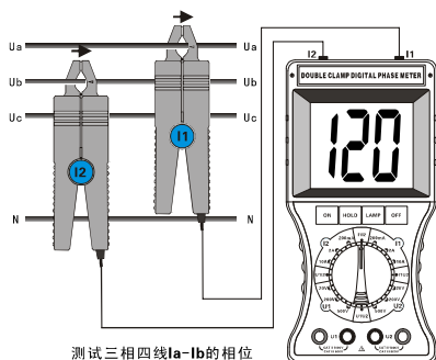
测试三相四线Ia-Ib的相位
